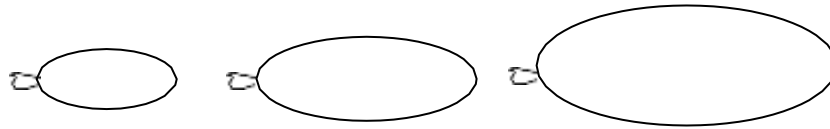
Gambar 70. Balon karet yang ditiup. (Sumber: https://www.google.com/search )
