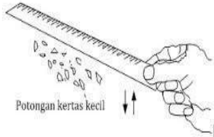
Gambar 17. Gaya Listrik Statis
