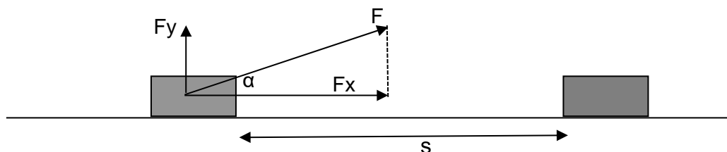
Gambar 28. Menggeser benda sejauh s dengan gaya F
