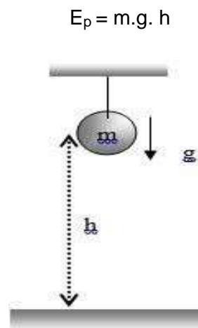
Gambar 27. Energi potensial
