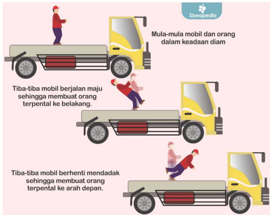
Gambar 22. Ilustrasi Hukum Newton I Sumber : https://www.siswapedia.com
