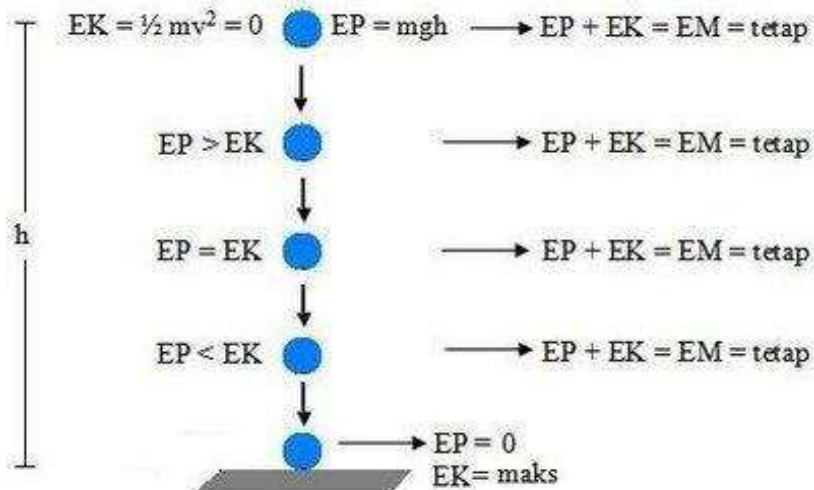
Gambar 26. Ilustrasi energi kinetik dan energi potensial Sumber : https://gagusketut.wordpress.com/
